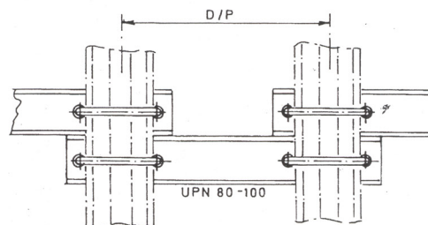
TRESILLONES UNION ABARCON INVERTIDO AL TRASPOLILLO (T.U.A.) 80/100-INV-T
