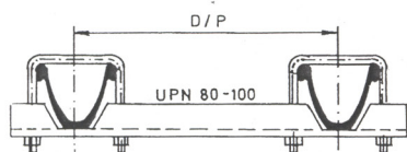
TRESILLONES UNION ABARCON (T.U.A.) 80/100
