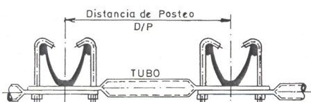
TRESILLONES UNION GANCHO (T.U.G.) T
