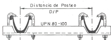
TRESILLONES UNION GANCHO (T.U.G.) 80/100
