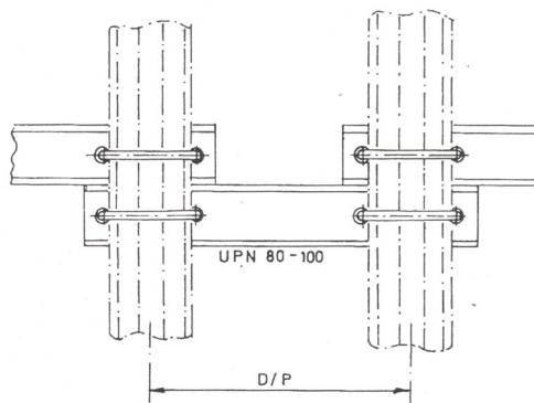
TRESILLONES UNION ABARCON (T.U.A.) 80/100
