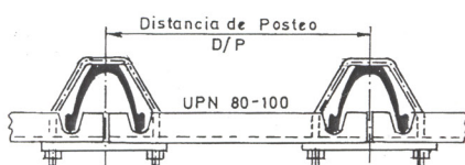
TRESILLONES UNION ABARCON INVERTIDO ALINEADO (T.U.A.) 80/100-INV-A
