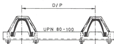
TRESILLONES UNION ABARCON INVERTIDO AL TRASPOLILLO (T.U.A.) 80/100-INV-T
